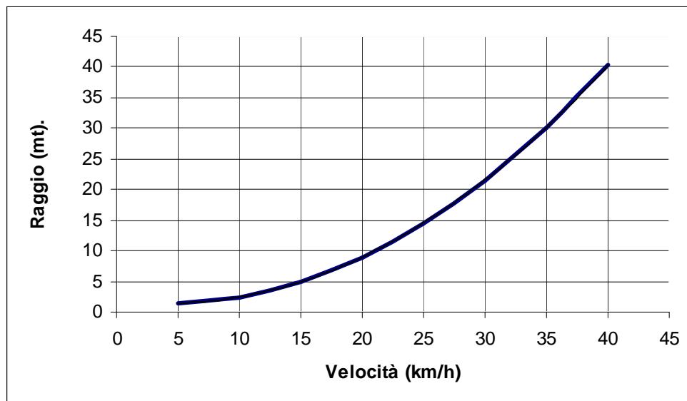
Fig. 2.1 Raggi minimi di curvatura in funzione della velocità di progetto 5
