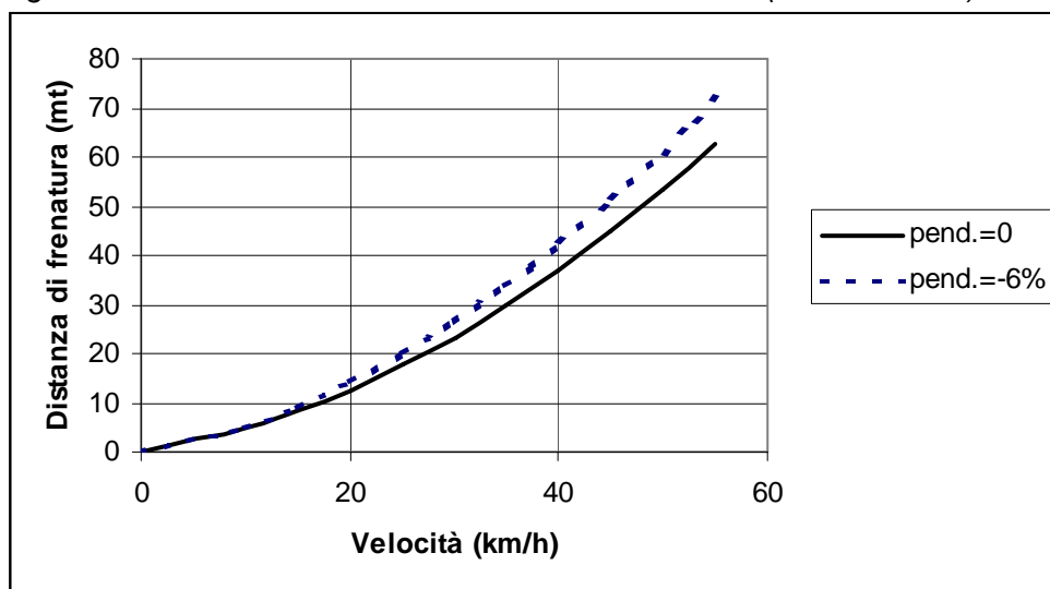
Fig.2.2 Distanza di frenatura in funzione della velocità (asfalto umido) 6
