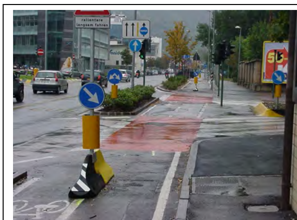
Esempio di continuazione della pista attraverso l'intersezione, realizzata con una banda colorata (Bolzano)
